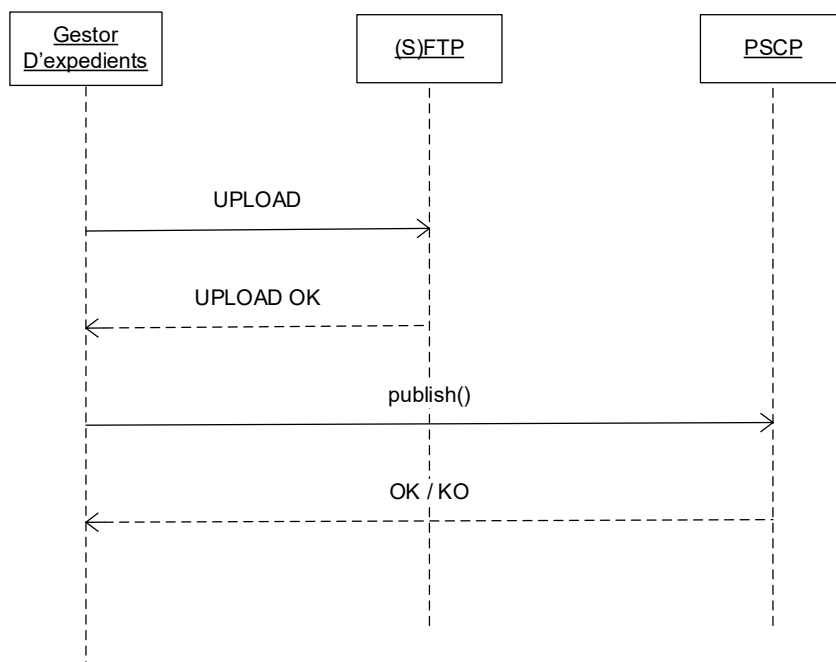
Diagrama de seqüència corresponent al procés d'enviament d'arxius
